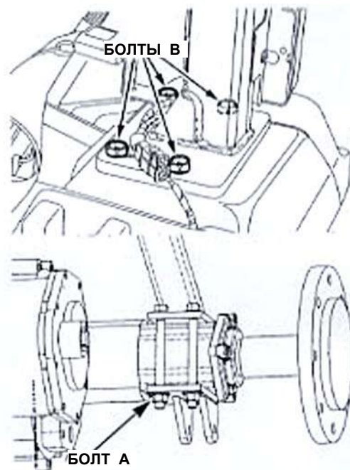
Рис. 66. Крепежные болты и гайки рамы ROPS
