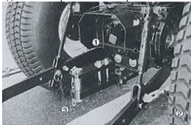
Рис. 33. Регулировка сцепки с тремя контактами
