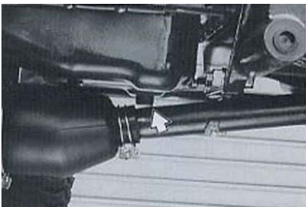
Рис. 51. Пробка слива моторного масла
