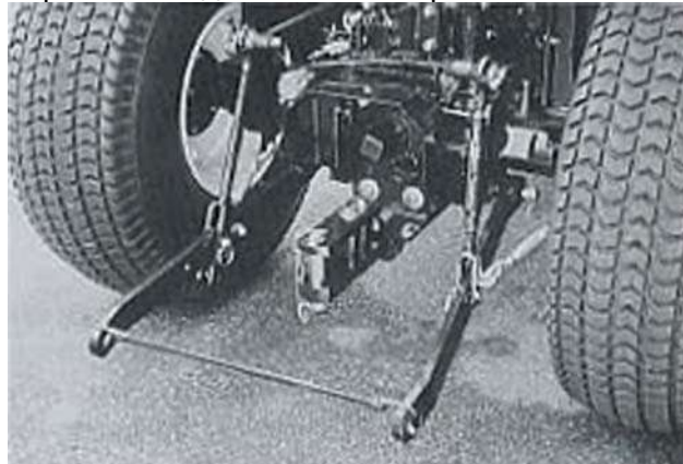
Рис. 32. Трехконтактная сцепка
