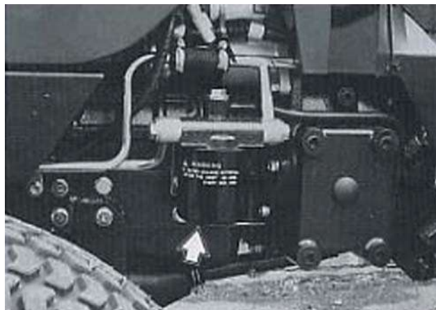
Рис. 58. Гидравлический масляный фильтр – ГСТ.
