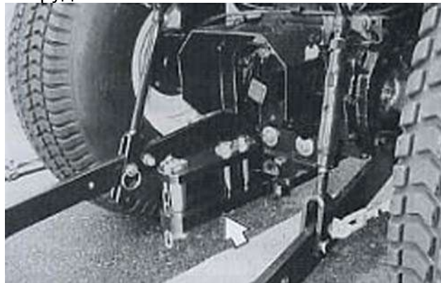
Рис. 29. Буксирная сцепка
