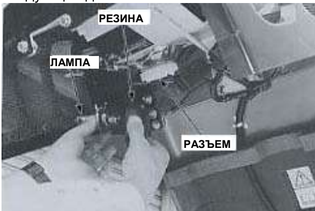
Рис. 74. Разъем фары
