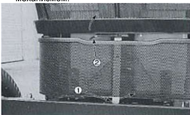
Рис. 30. Защелки капота
